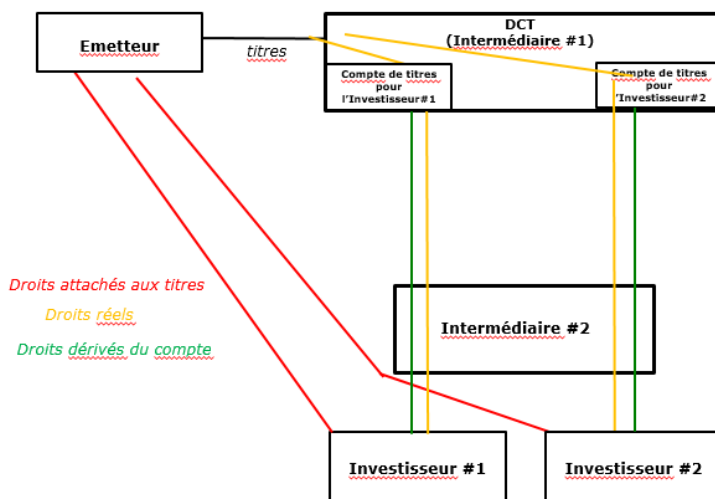
Schéma 51-1: Système transparent dans lequel les titres de l'investisseur sont détenus dans un compte auprès du DCT
